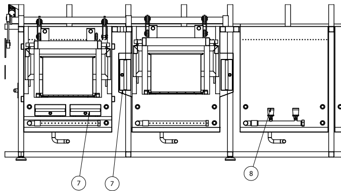
D-D ( 1 : 10 )
