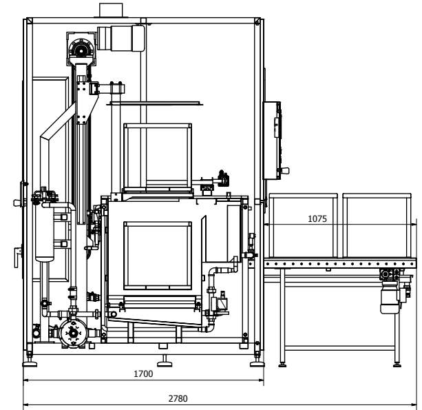
A-A (1 : 13)
